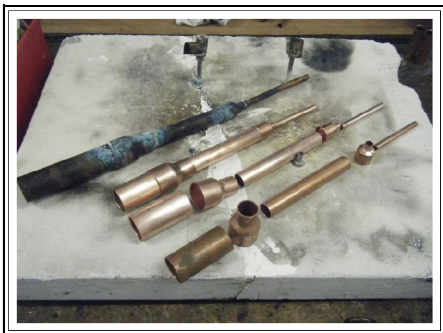
Pièces réalisées pour l'habilitation brasage
