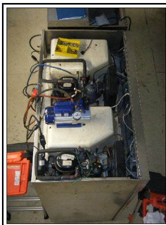
Armoire froid 2 portes – compresseur numéro 1 en cours de tirage au vide
