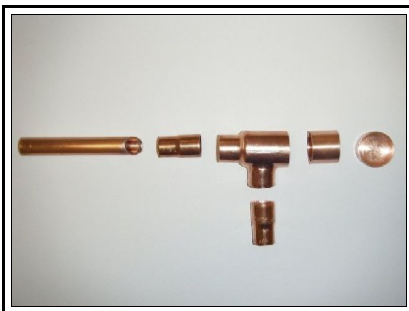
Piège à huile – les éléments avant assemblage
