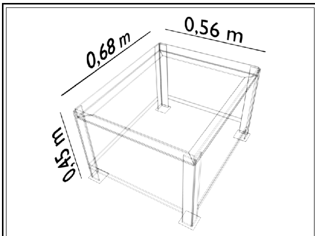
Bâti métallique pour machine à glace - dimensions
