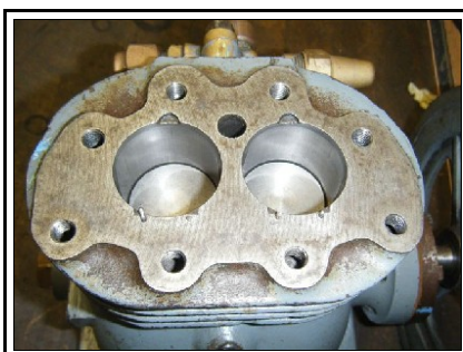
Compresseur à piston
