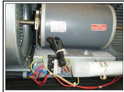
Moteur des ventilateurs tangentiels
