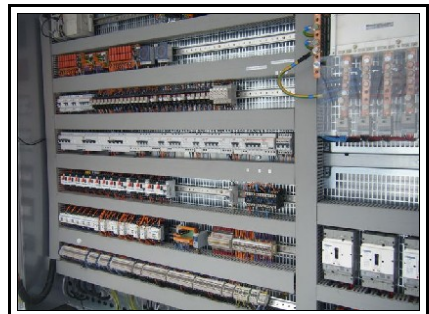
Armoire électrique
