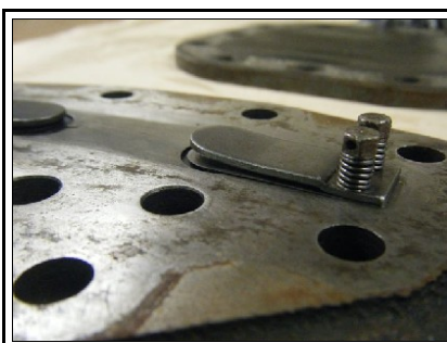
Compresseur à piston, plaque à clapet, détail d'un clapet HP
