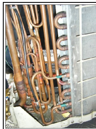
Détail de la tubulure de l'unité extérieure
