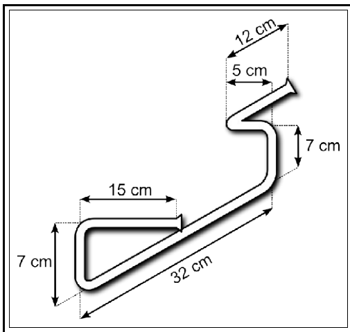
Cintrage et dudgeonnage à réaliser
