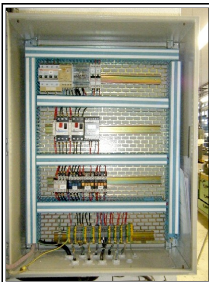
Intérieur de l'armoire électrique
