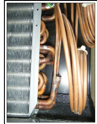
Distributeur à l'entrée de l'évaporateur
