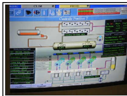
Un des écrans pour le contrôle et la surveillance du système
