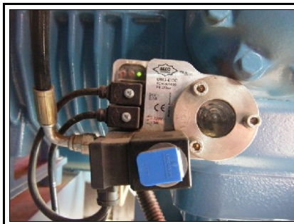
Régulateur de niveau d'huile
