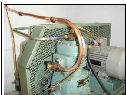
Détail du compresseur et des tubulures
