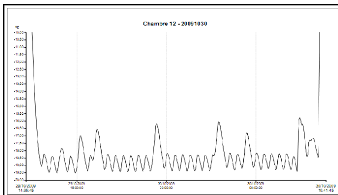
Chambre froid négatif, historique des températures, avec dégivrages
