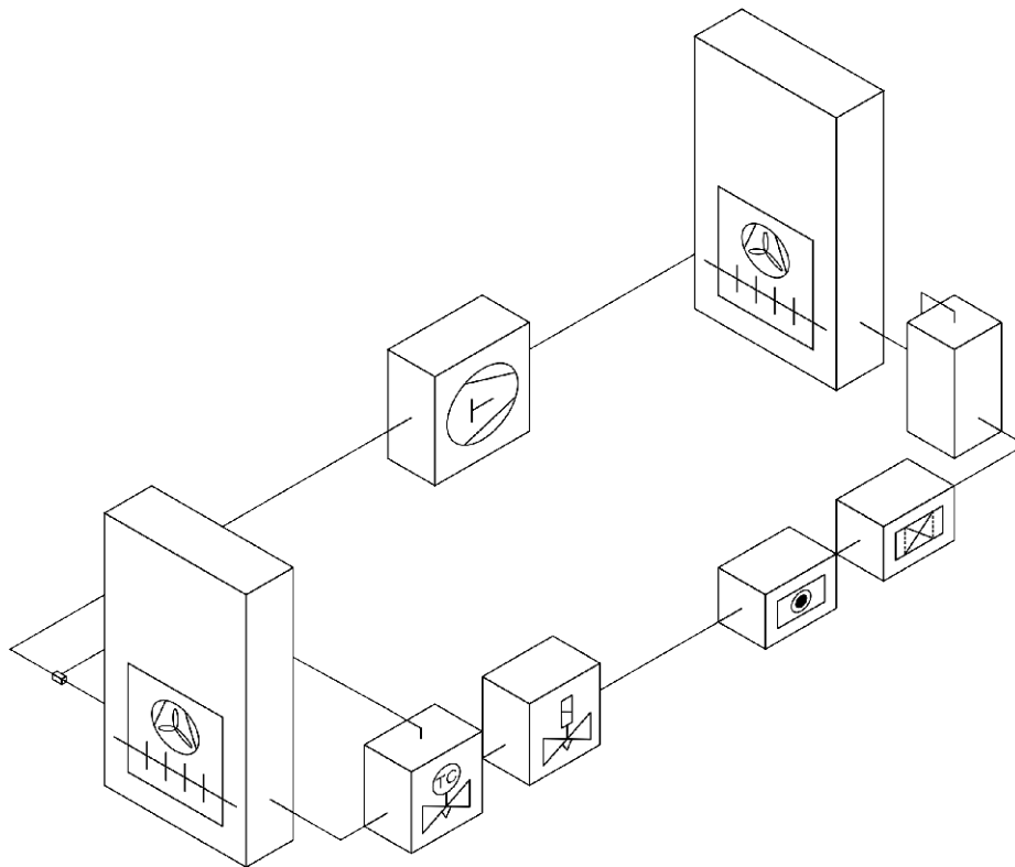
Schéma isométrique d'un circuit frigorifique simplifié
