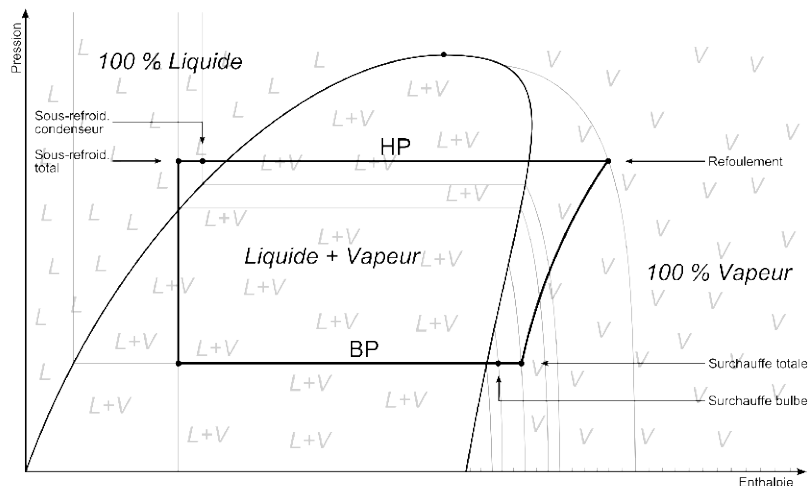
Diagramme enthalpique (points remarquables)
